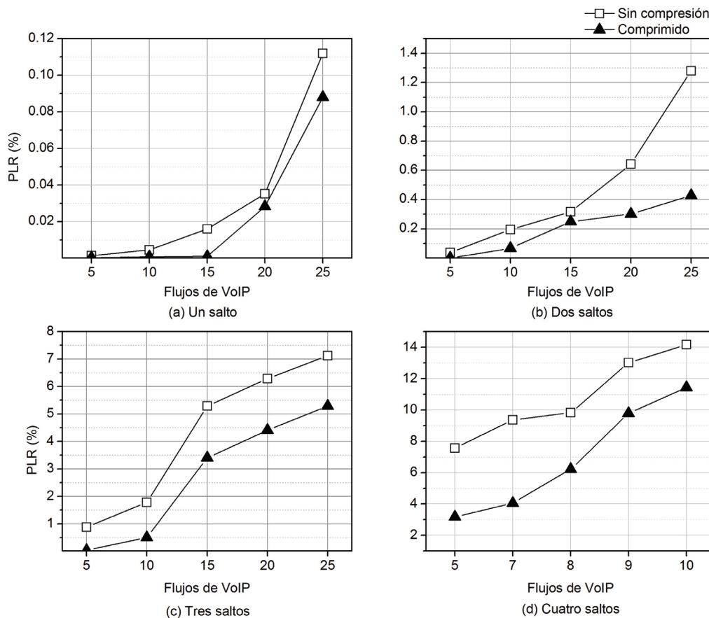
Figura 8 Tasa de pérdida de paquetes
